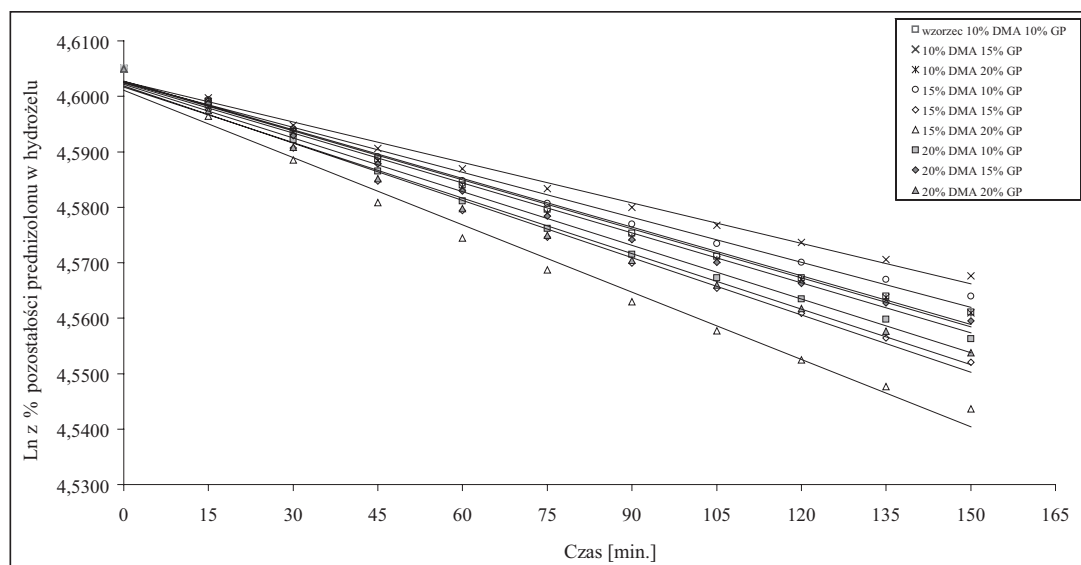
Ryc. 1. Wpływ wzrastających stężeń DMA na proces uwalniania prednizolonu z hydrożeli zawierających 0,5% substancji leczniczej
