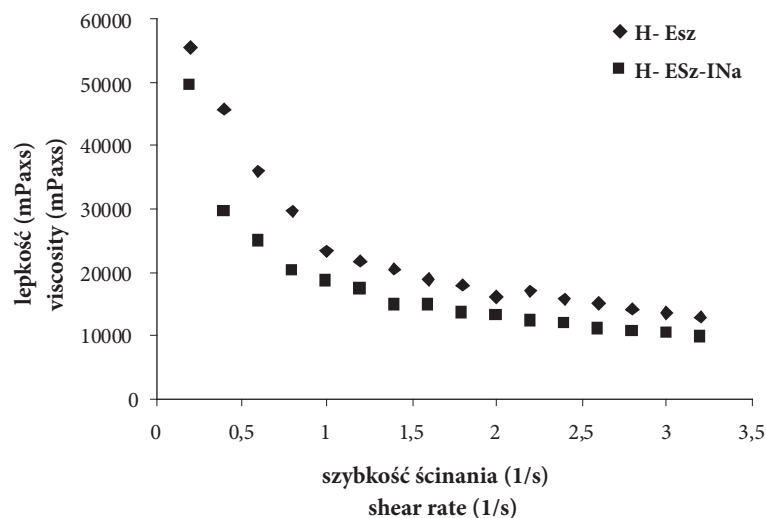
Ryc. 3. Krzywe lepkości hydrożeli z ekstraktem z szałwii
